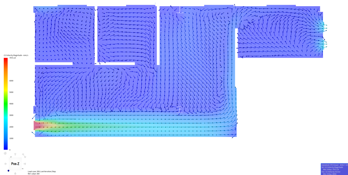
Figura 2: Campo de magnitud de velocidad en el plano horizontal (vista +Z). Simulación CFD (Autodesk CFD 2020); escala 0–7973 mm/s. Flujo desde la impulsión inferior izquierda hacia las rejillas del lateral derecho, con vórtices en los recintos secundarios.
