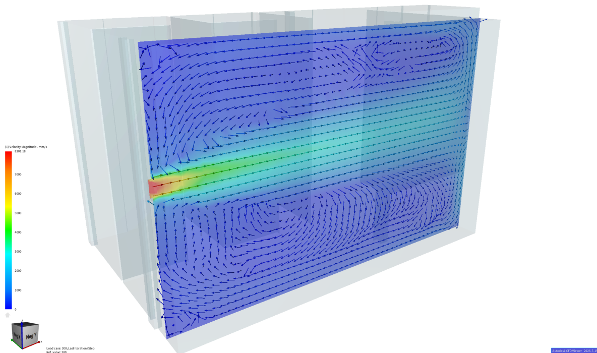
Figura 1: Campo de magnitud de velocidad en el plano vertical longitudinal (vista –Y). Simulación CFD (Autodesk CFD 2020); escala 0–8201 mm/s ( \approx 8,2 \text{ m/s} en el máximo), consistente con la velocidad de impulsión de diseño. Se aprecia la inyección lateral y la recirculación en las zonas periféricas del recinto.
